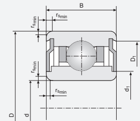
X-2Zシリーズ
