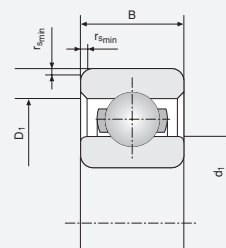
60/62シリーズ
