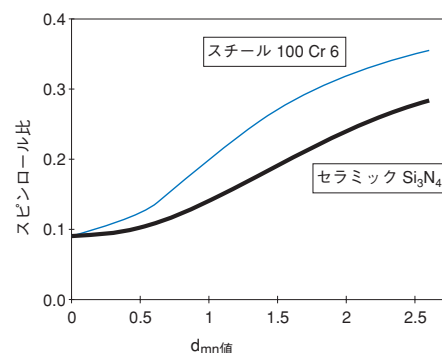
図-1 dmn値とスピンロール比
